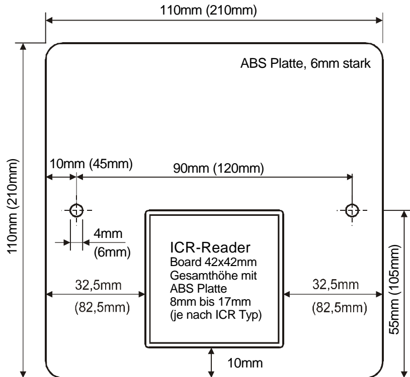
Abmessungen ICR-Reader mit Antenne S1 (abweichende Werte für S2 in Klammern)
